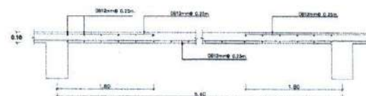
รูปตัดทางด้านขวา (S12)
