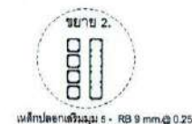
เหล็กปลอกเสริมรุ่น 5 - RB 9 mm @ 0.25
