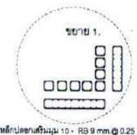
เหล็กปลอกเสริมขนาด 10 - RB 9 mm. @ 0.25
