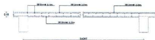
รูปตัดทางด้านขึ้น
